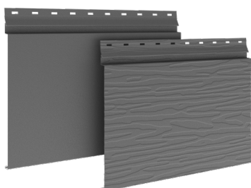
СКАНДИНАВСКИЙ БРУС «МОДЕРН» ШИРОКИЙ Одноsegmentная панель с шириной видимой части 206 мм
